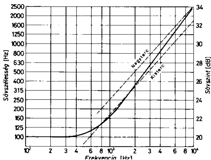
7. ábra A kritikus sáv szélesség változása a sávközepi frekvencia függvényében
