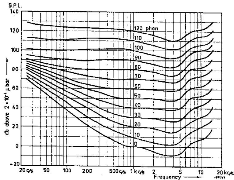
4. ábra. Azonos hangosságintű görbék Fletcher-Munson szerint
